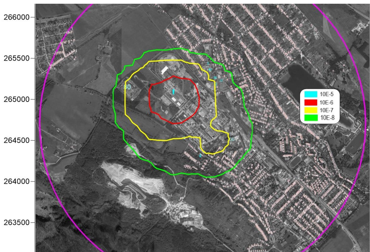
A Szenáriók egyéni összesített izokockázati térképe
