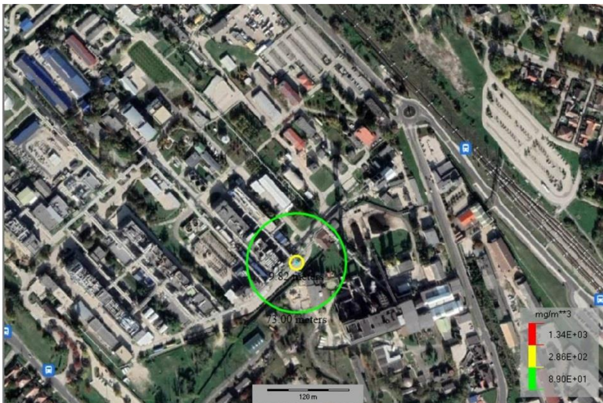
Metanszulfonil-klorid kikerülésének izokoncentrációs görbéi
